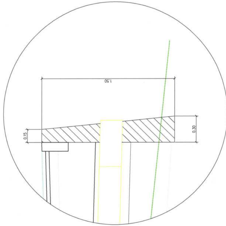
IZLAZNA GLAVA PROPUSTA Ø250
