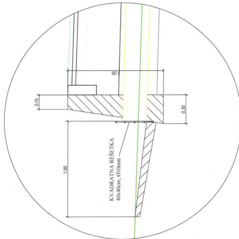
ULAZNA GLAVA PROPUSTA Ø250
