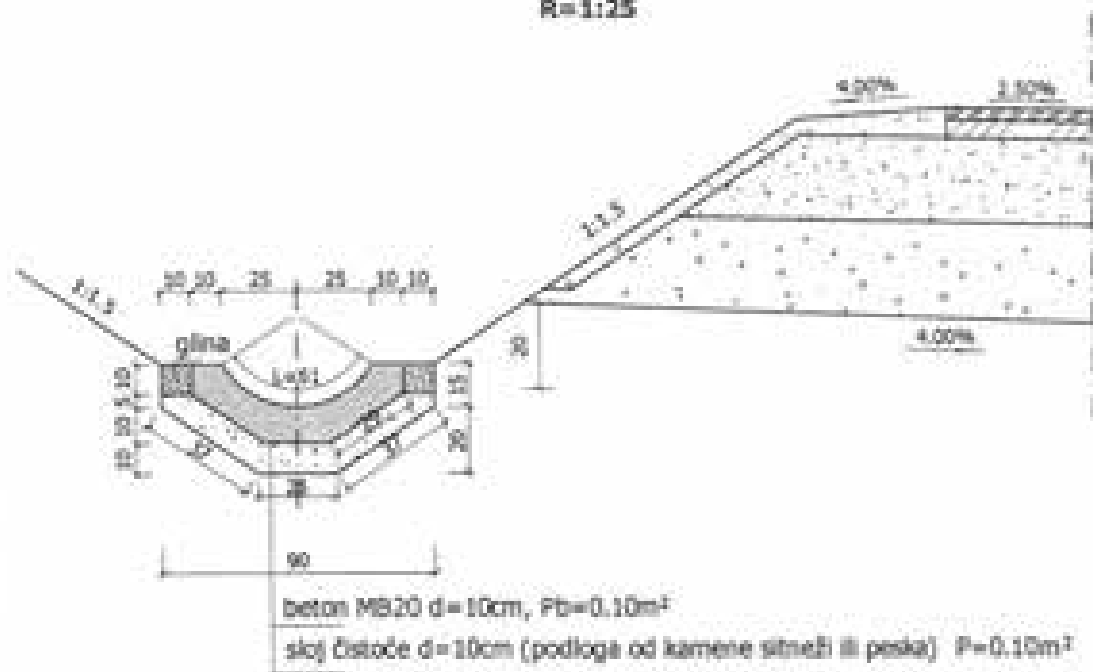
Detalj "A" za podužni nagib kanala >5.0% R=1:25
