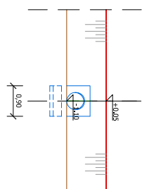
Изглед улаза пропуста R = 1:50
