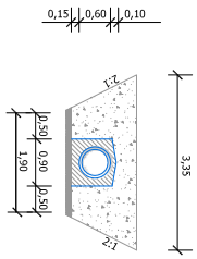
Штрључани кљин R=1:50
