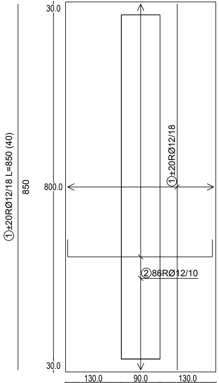
Temelj mosta d.zona
