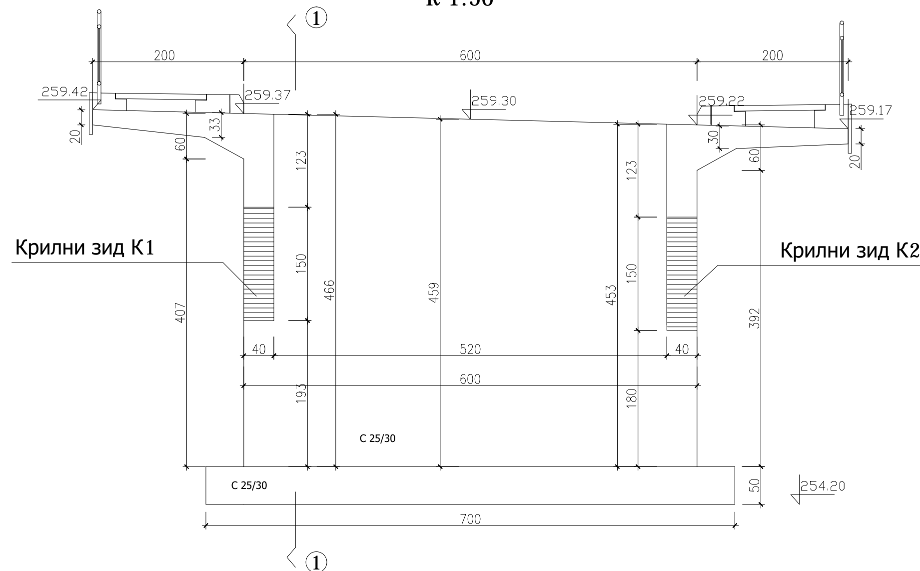
КАРАКТЕРИСТИЧАН ПОПРЕЧНИ ПРЕСЕК РАСПОНСКЕ КОНСТРУКЦИЈЕ R 1:50
