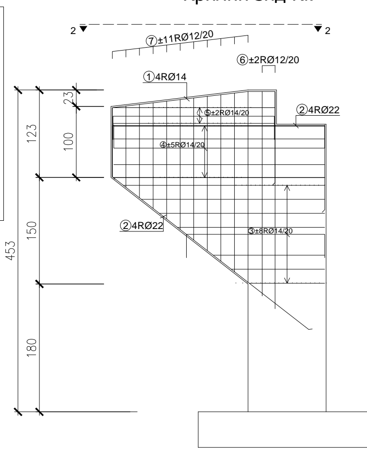
Крилни зид К2
