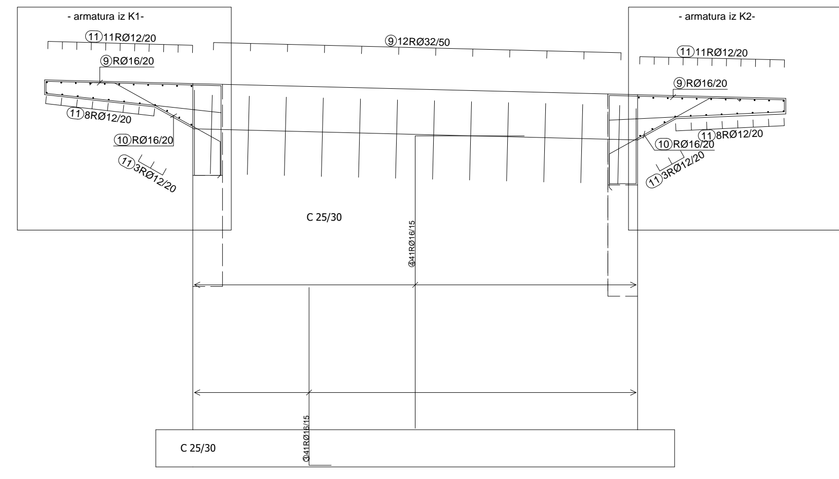
Крилни зид К1
