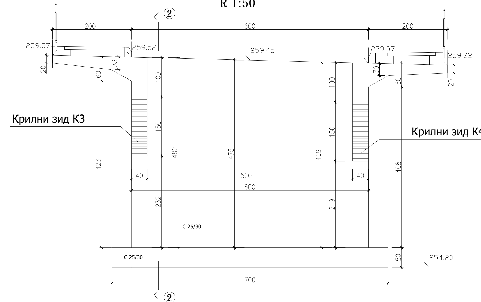
ПОПРЕЧНИ ПРЕСЕК СТУБА С2 R 1:50
