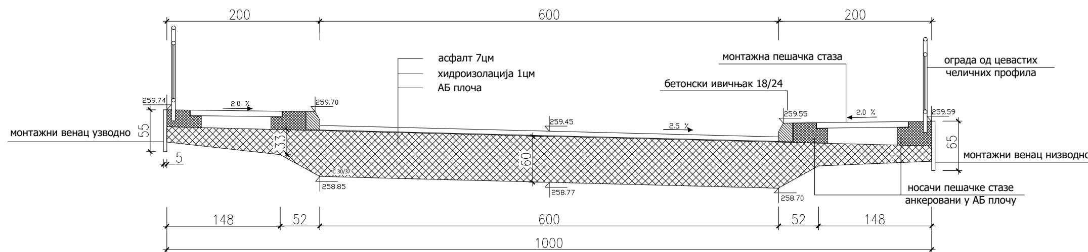
КАРАКТЕРИСТИЧАН ПОПРЕЧНИ ПРЕСЕК РАСПОНСКЕ КОНСТРУКЦИЈЕ R 1:50
