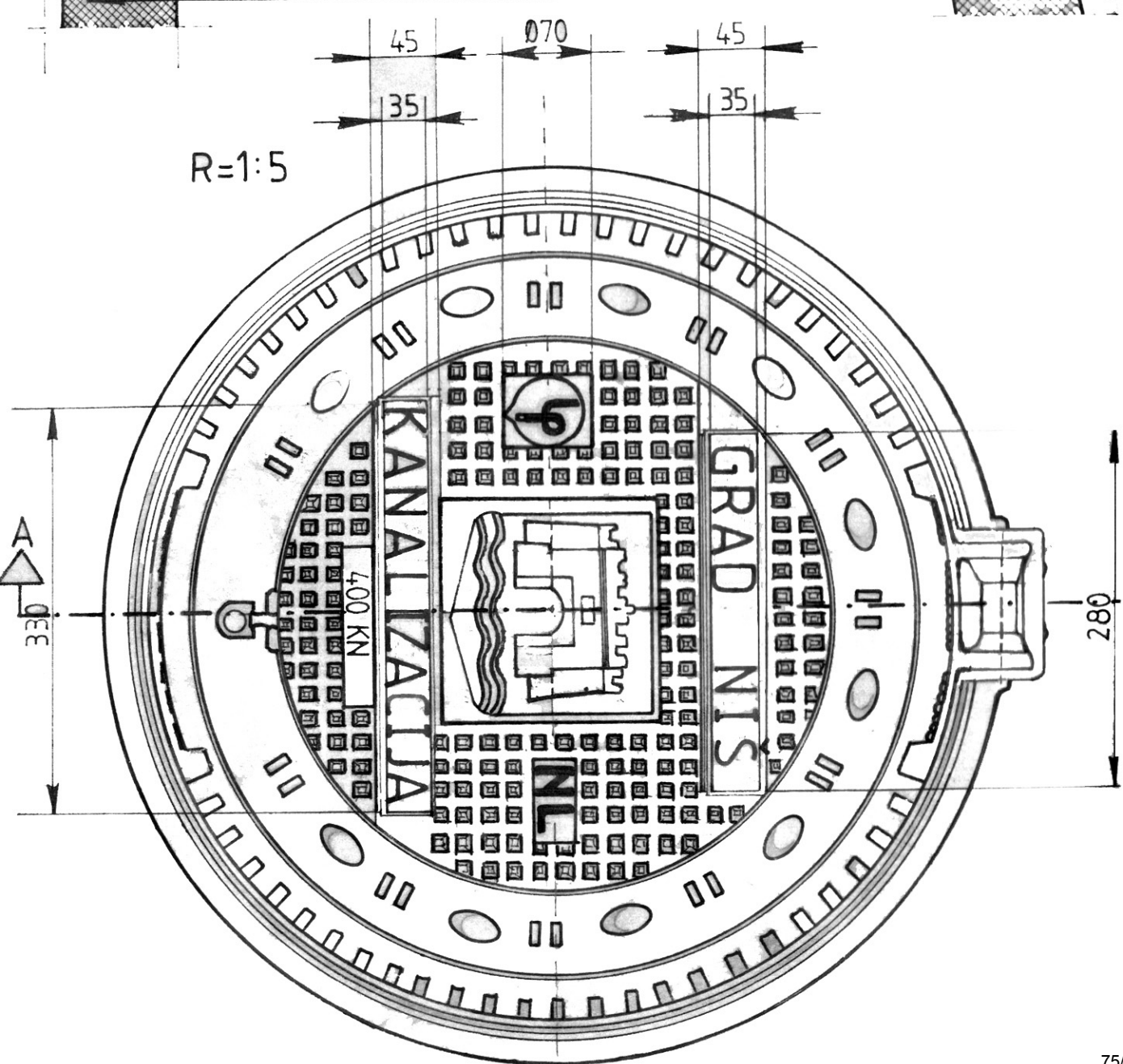
OSNOVA ŠAHTNOG POKLOPCA
