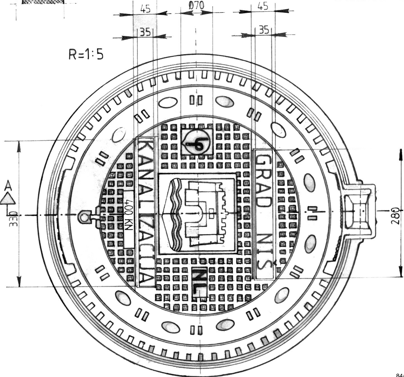
OSNOVA ŠAHTNOG POKLOPCA
