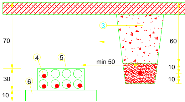
paralelno vođenje energetskih i PTT kablova
