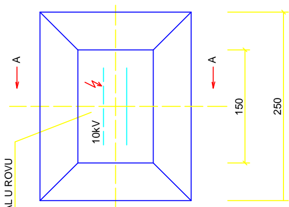
IZGLED ODOZGO
