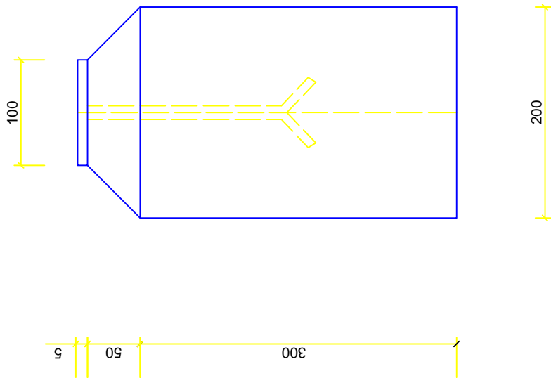
PRESEK A-A
