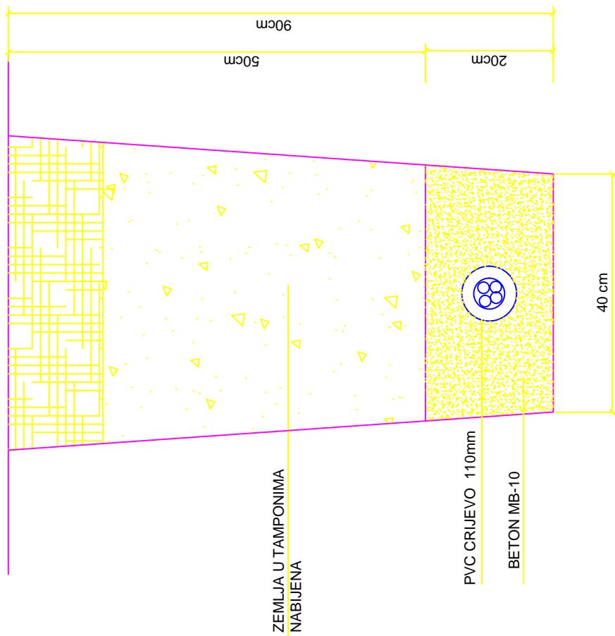
DETALJ KABLOVSKOG PROLAZA ISPOD SAOBRACAJNICE
