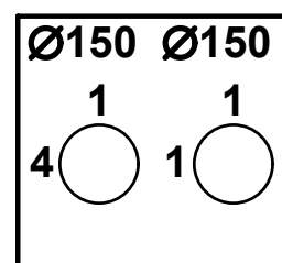
Kablovska kanalizacija u 1 redu sa 4 otvora Ø100 i jednim Ø150
