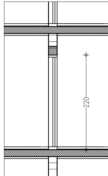
presek
