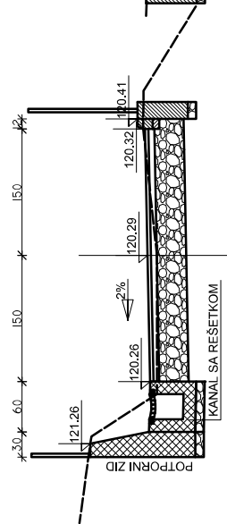
PROFIL 3 0+020.00
