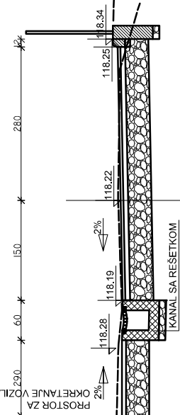
PROFIL 6 0+042.89
