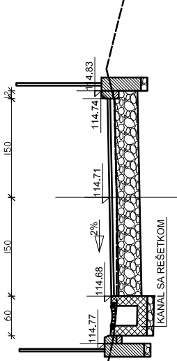
PROFIL 8 0+066.77
