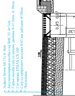
Деталј Гајгеровог сливника P=1:25
