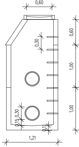
Деталј малог ивичњака P=1:10
