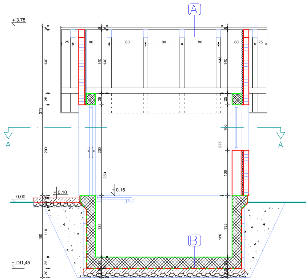
PRESEK I-I
