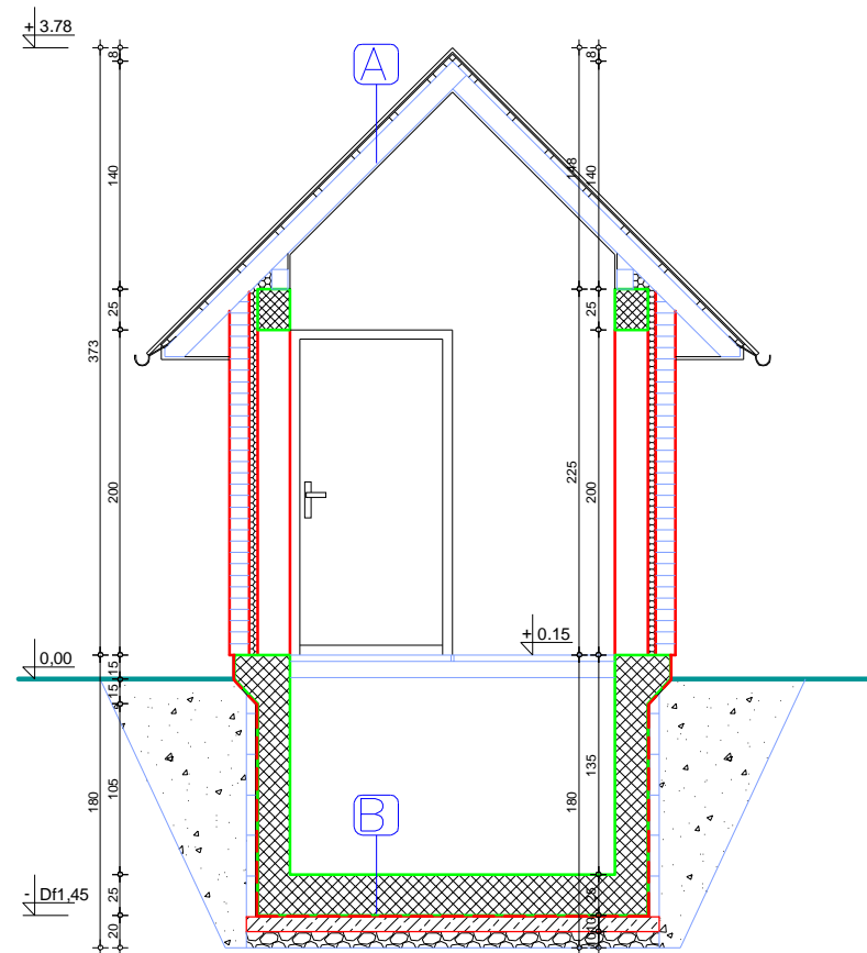
PRESEK II-II
