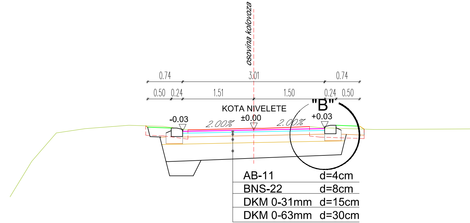
KARAKTERISTIČNI POPREČNI PROFIL OSOVINE SAOBRAĆAJNICE CL-1 NA STACIONAŽI km 0+435.31
