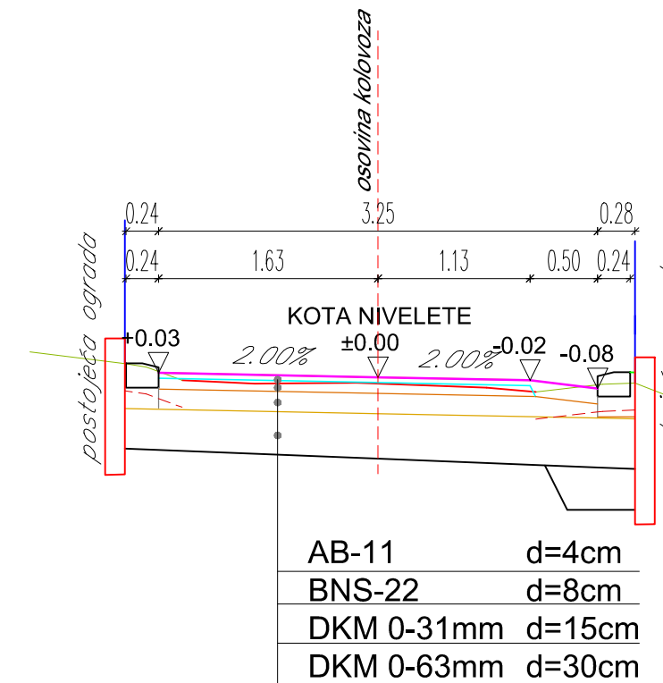
KARAKTERISTIČNI POPREČNI PROFIL OSOVINE SAOBRAĆAJNICE CL-2 NA STACIONAŽI km 0+060.00
