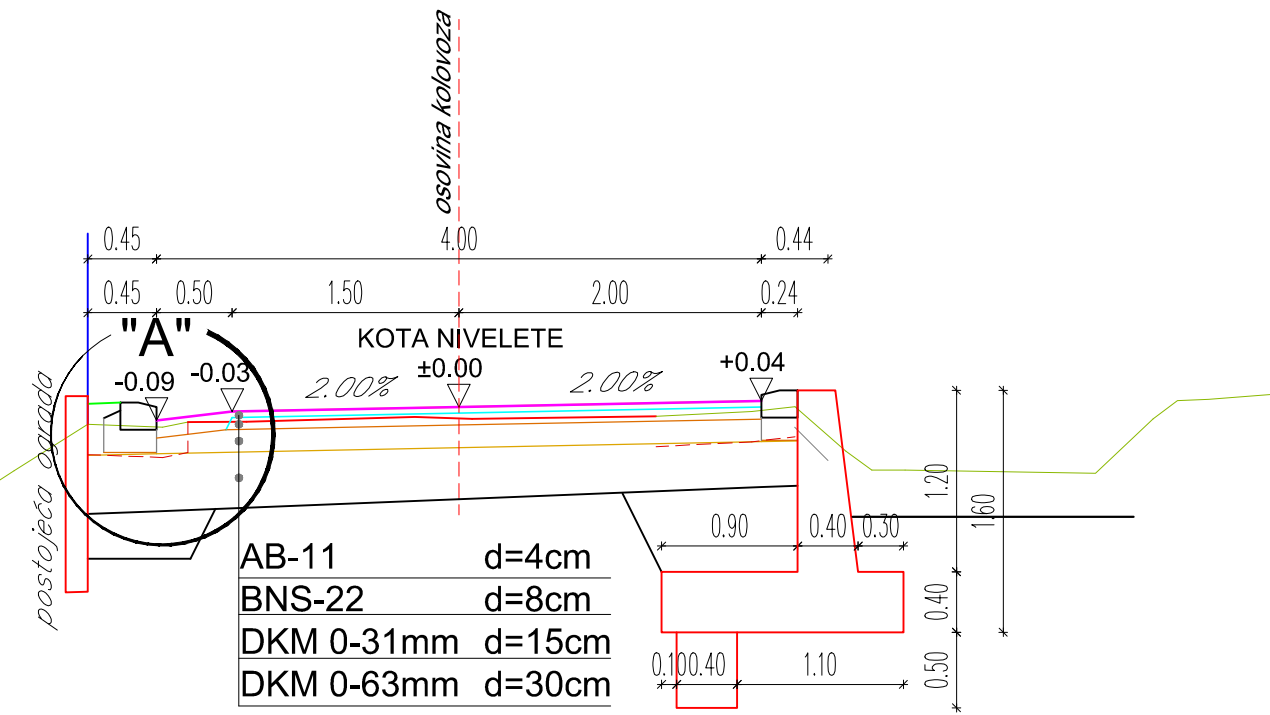
KARAKTERISTIČNI POPREČNI PROFIL OSOVINE SAOBRAĆAJNICE CL-1 NA STACIONAŽI km 0+070.00
