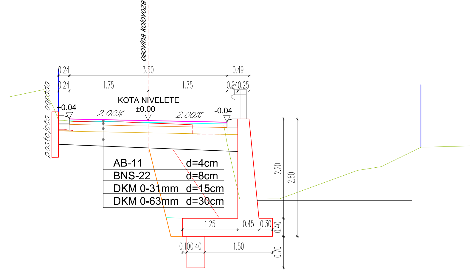
KARAKTERISTIČNI POPREČNI PROFIL OSOVINE SAOBRAĆAJNICE CL-1 NA STACIONAŽI km 0+385.93
