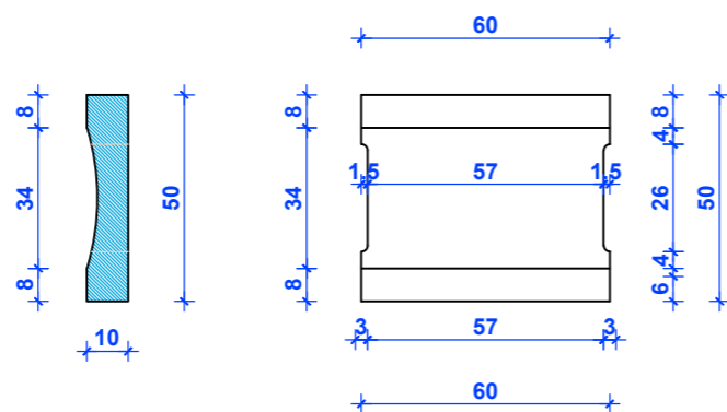
rigola dimenzija 60/50/10cm
