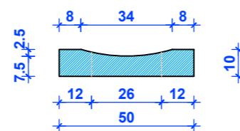
poprecni presek kroz rigolu
