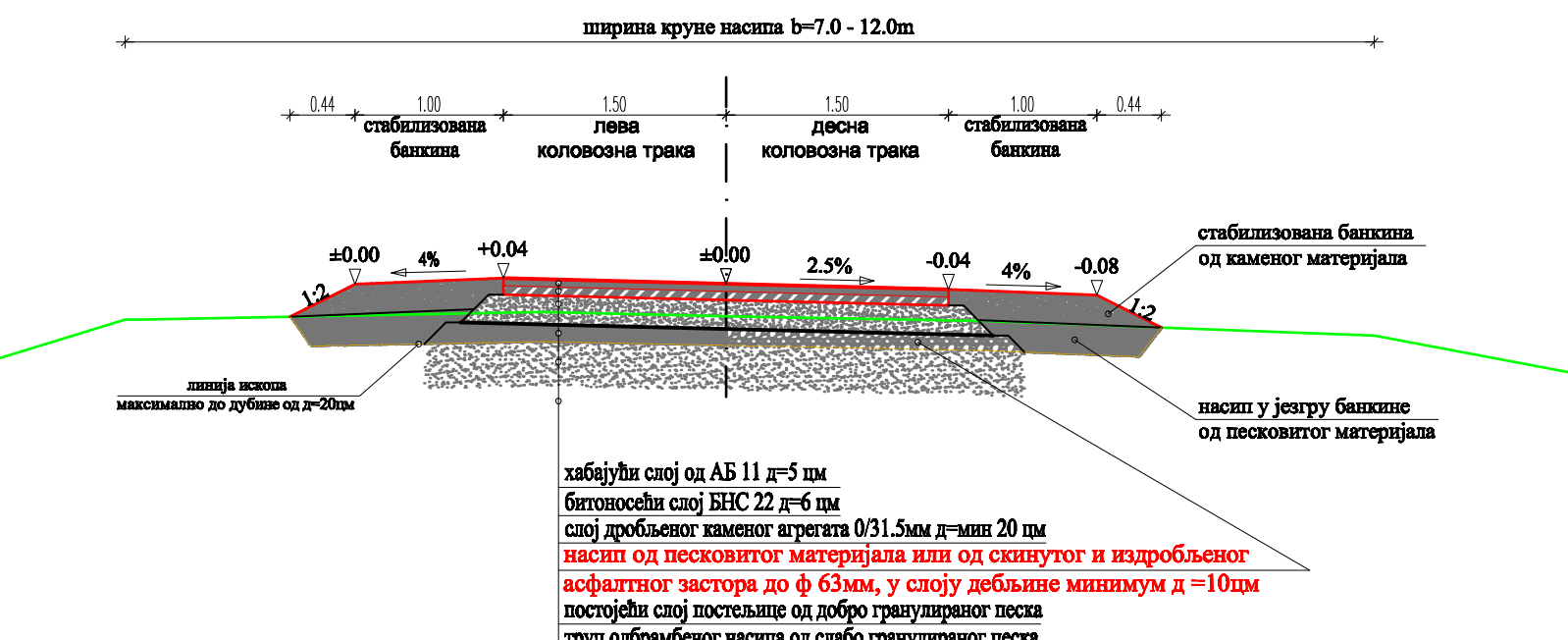
НОРМАЛАН ПОПРЕЧНИ ПРОФИЛ ПРОЈЕКТОВАНОГ РЕШЕЊА РЕКОНСТРУКЦИЈЕ ПУТА СА КОЛОВОЗНОМ КОНСТРУКЦИЈОМ
