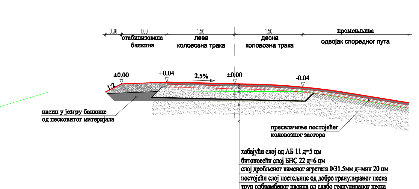
НОРМАЛАН ПОПРЕЧНИ ПРОФИЛ ПРОЈЕКТОВАНОГ РЕШЕЊА РЕКОНСТРУКЦИЈЕ ПУТА НА МЕСТУ УЛИВА СПОРЕДНОГ ПУТА
