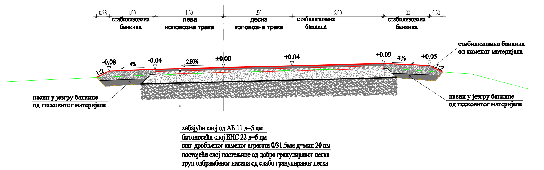
НОРМАЛАН ПОПРЕЧНИ ПРОФИЛ ПРОЈЕКТОВАНОГ РЕШЕЊА РЕКОНСТРУКЦИЈЕ ПУТА СА ПРОЈЕКТОВАНОМ МИМОИЛАЗНИЦОМ
