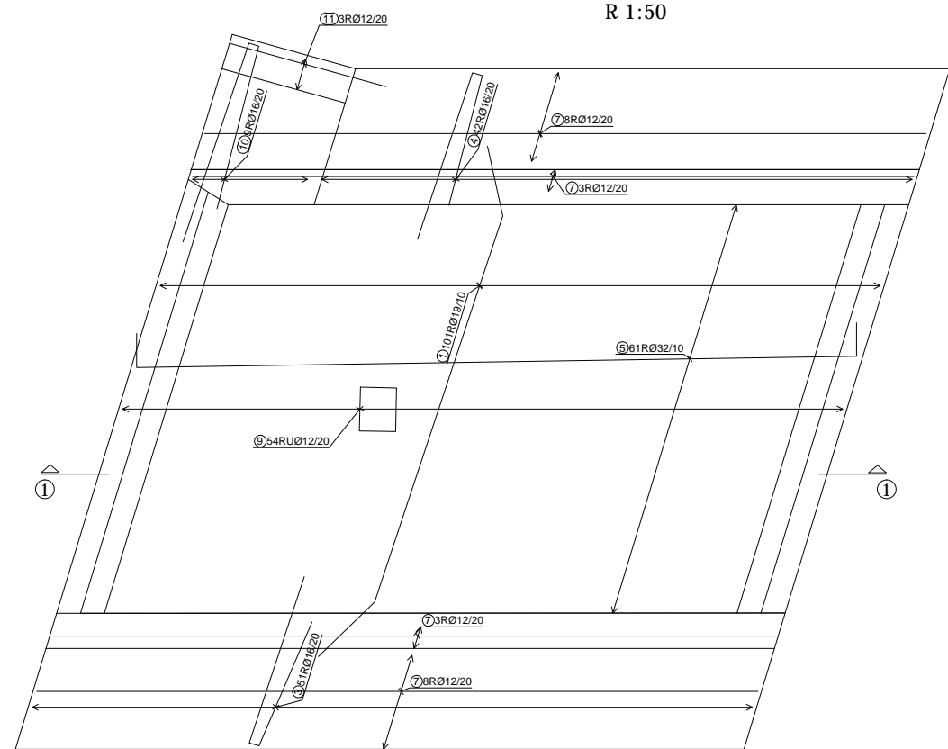
ПЛАН АРМАТУРЕ КОЛОВОЗНЕ ПЛОЧЕ ДОЊА ЗОНА R 1:50
