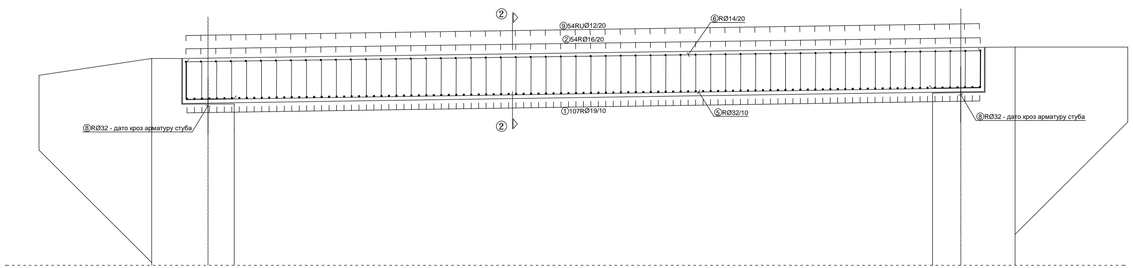
ПЛАН АРМАТУРЕ КОЛОВОЗНЕ ПЛОЧЕ ПОДУЖНИ ПРЕСЕК 1-1 R 1:50
