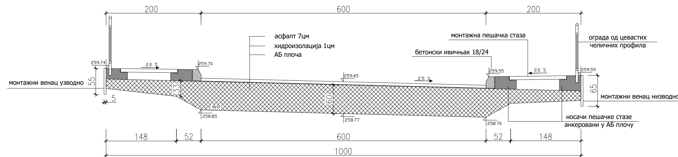
КАРАКТЕРИСТИЧАН ПОПРЕЧНИ ПРЕСЕК РАСПОНСКЕ КОНСТРУКЦИЈЕ R 1:50
