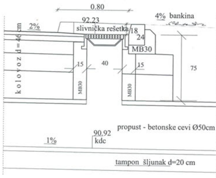
detalj slivničkog šahta R 1:25
