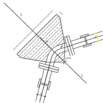
изглед одозго
