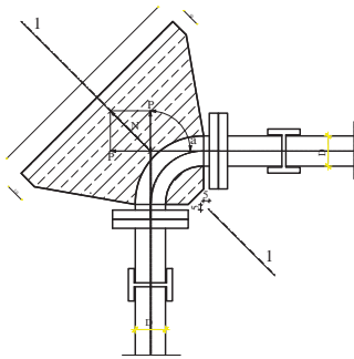
ПРЕСЕК 1-1
