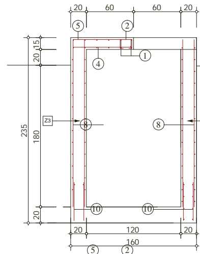
PRESEK 2-2
