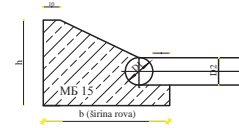
ПРЕСЕК 2-2
