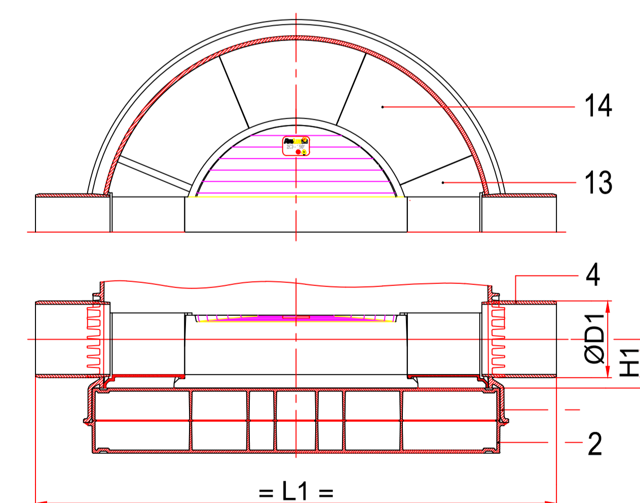
Шахт - колектор вратила 1000 и купе Ø630
