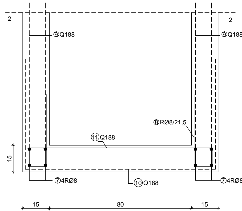
PRESEK 2 - 2 ZIDOVİ IZLIVA
