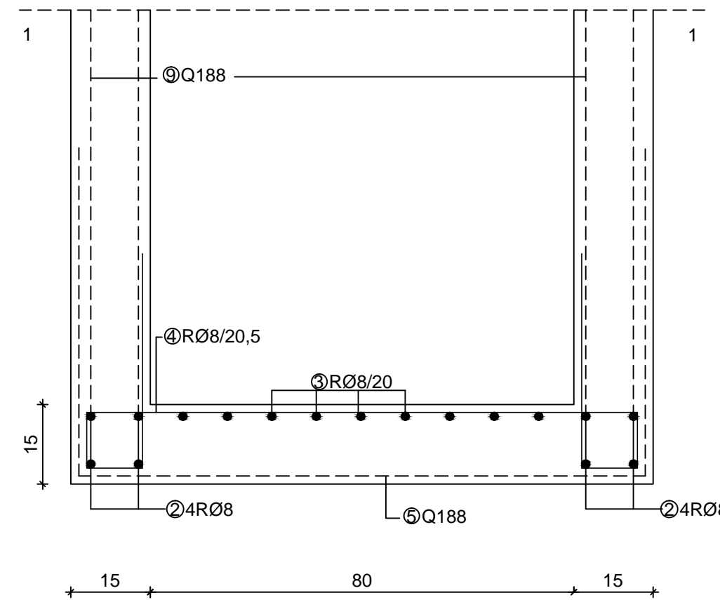
PRESEK 1 - 1 DNO IZLIVA I ZIDOVİ
