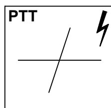
Oznaka za ukrštanje kabla sa TT vodom
