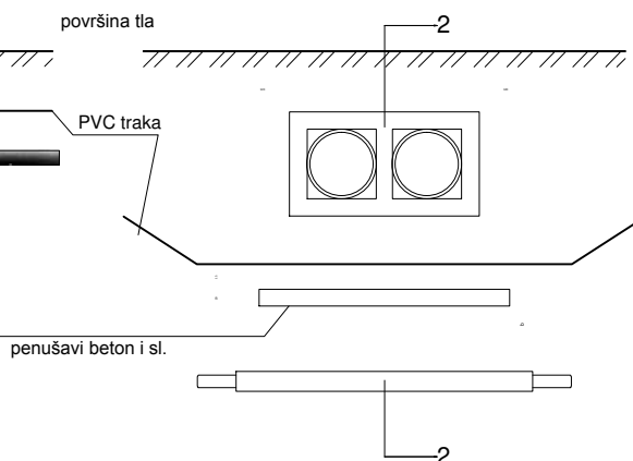
PRESEK 2 - 2
