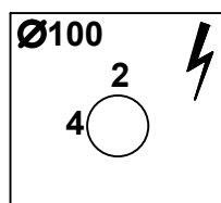
Kablovska kanalizacija Ø100 u 2 reda po 4 otvora
