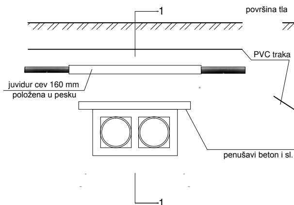
PRESEK 1 - 1
