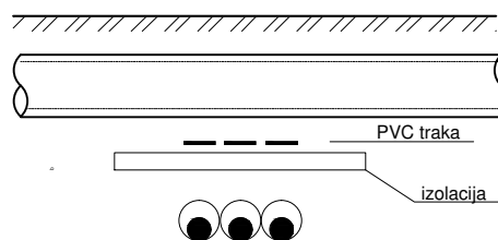
PRESEK 2 - 2
