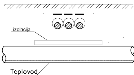
PRESEK 1 - 1
