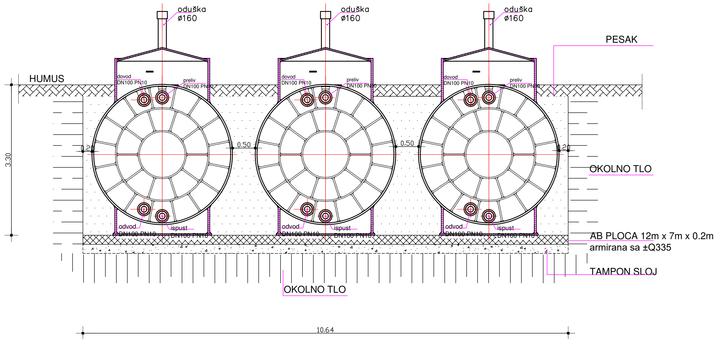
HORIZONTALNI REZERVOAT TIP "C" Ø3000x10800mm OD PEHD SA ZATVARAČNICOM
