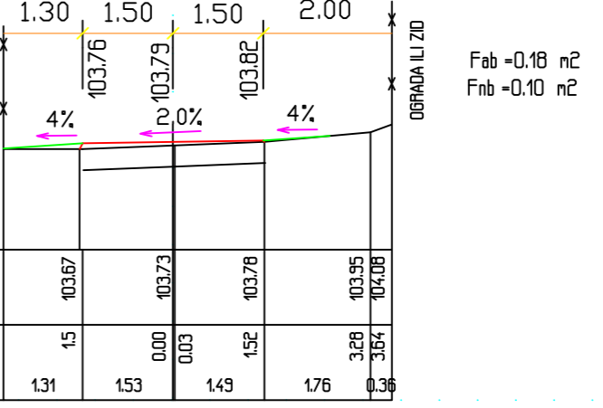
PROFIL 16: 0+402.89 RAZMERA 1:100
