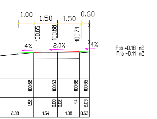
PROFIL 12: 0+316.08 RAZMERA 1:100
