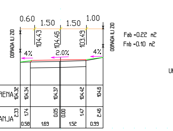
PROFIL 17: 0+411.82 RAZMERA 1:100
