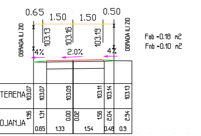
PROFIL 15: 0+393.27 RAZMERA 1:100
