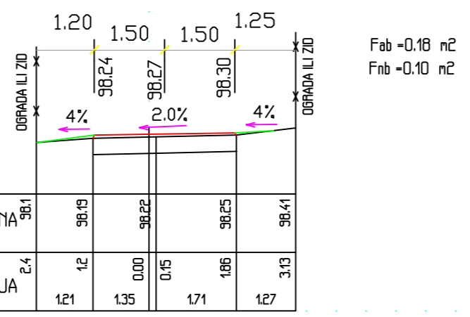
PROFIL 7: 0+180.80 RAZMERA 1:100
