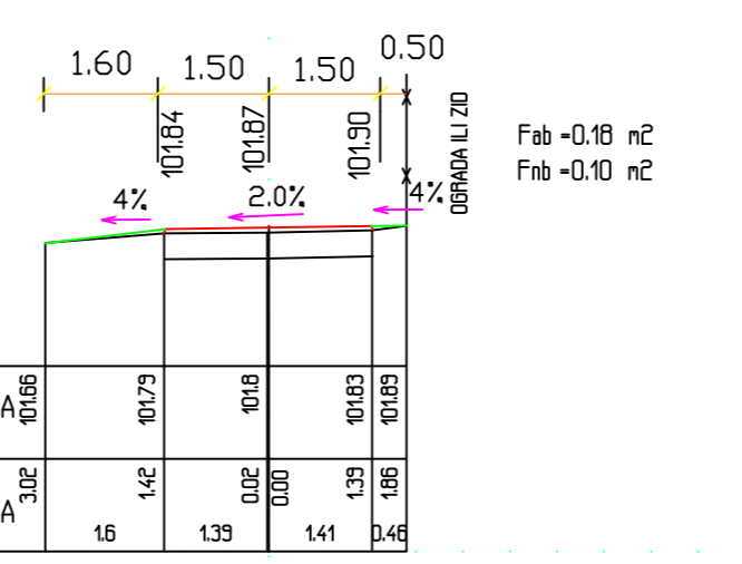
PROFIL 14: 0+360.46 RAZMERA 1:100
