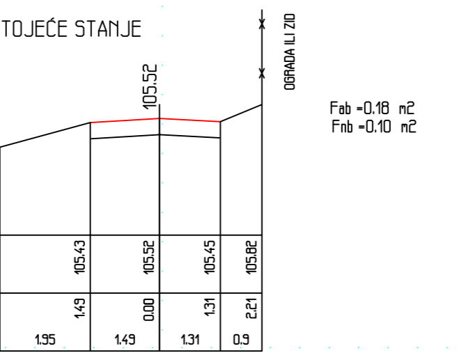
PROFIL 18: 0+421.57 RAZMERA 1:100
