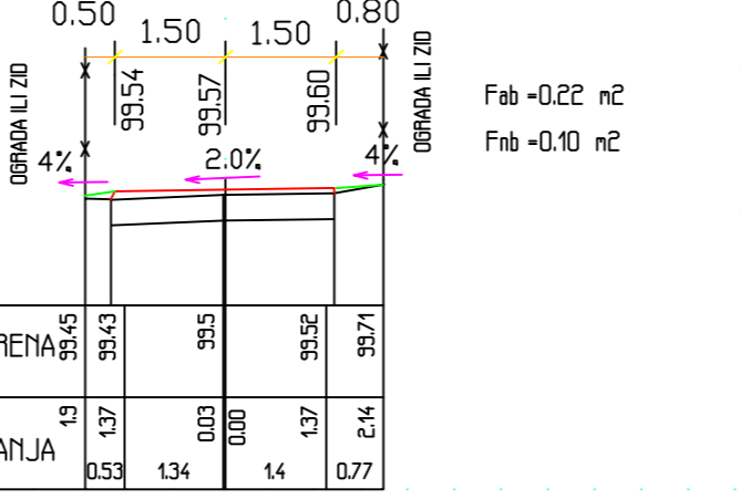
PROFIL 10: 0+274.55 RAZMERA 1:100
