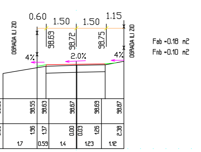
PROFIL 8: 0+213.87 RAZMERA 1:100
