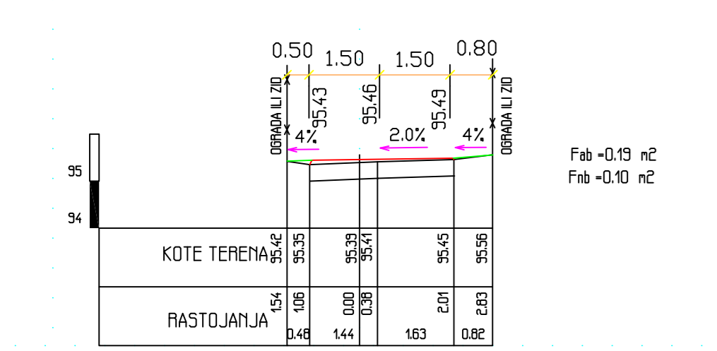
PROFIL 3: 0+055.62 RAZMERA 1:100
