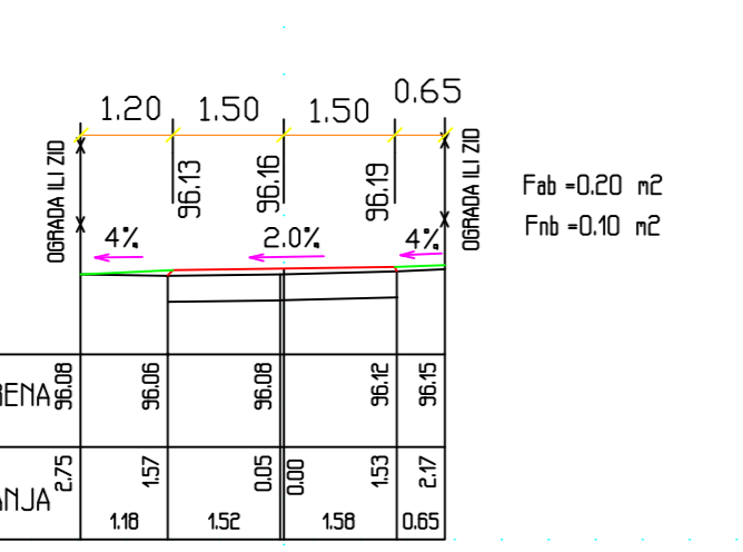
PROFIL 5: 0+103.80 RAZMERA 1:100
