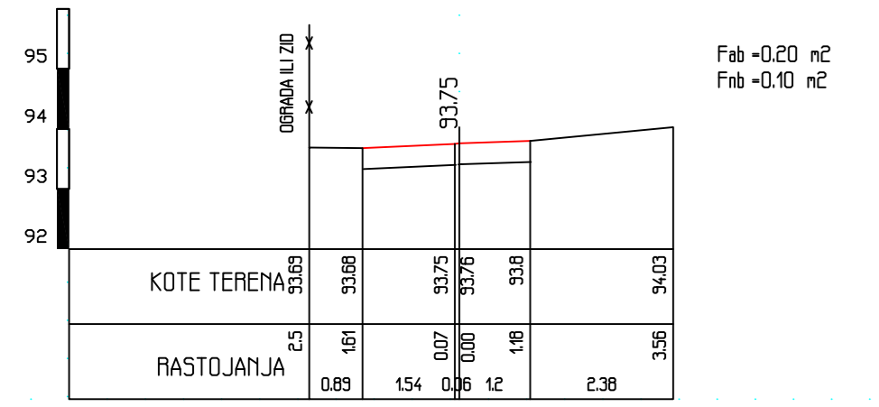
PROFIL 2: 0+030.74 RAZMERA 1:100
