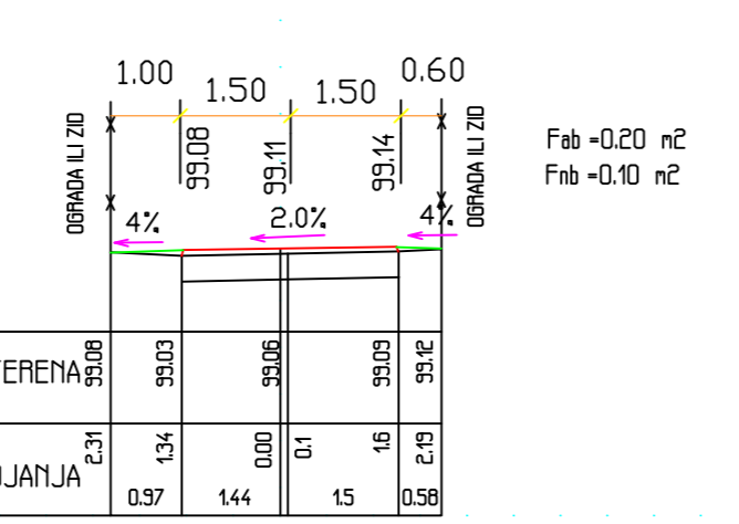
PROFIL 9: 0+241.62 RAZMERA 1:100
