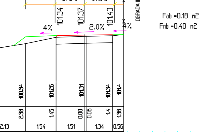
PROFIL 13: 0+342.80 RAZMERA 1:100
