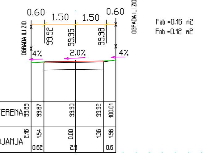
PROFIL 11: 0+288.74 RAZMERA 1:100
