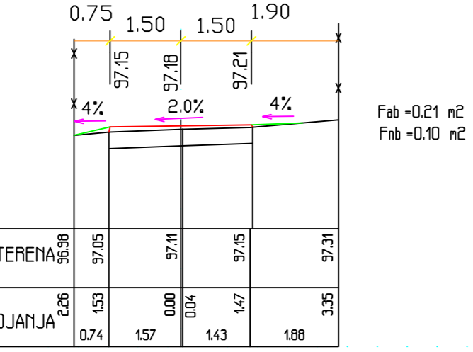
PROFIL 6: 0+145.58 RAZMERA 1:100
