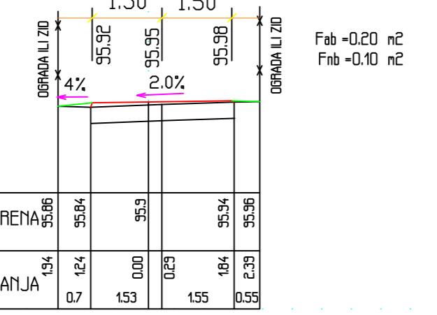
PROFIL 4: 0+082.17 RAZMERA 1:100
