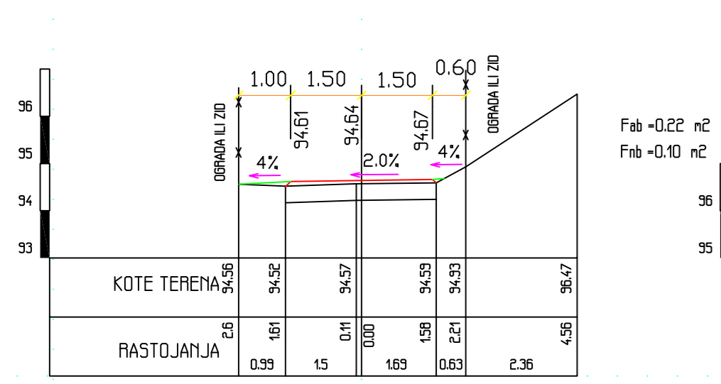
PROFIL 2: 0+030.74 RAZMERA 1:100
