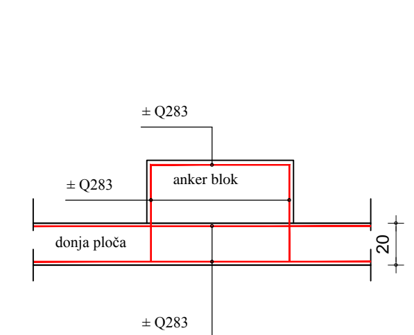
SPOJ DONJE PLOČE I ANKER BLOKA
