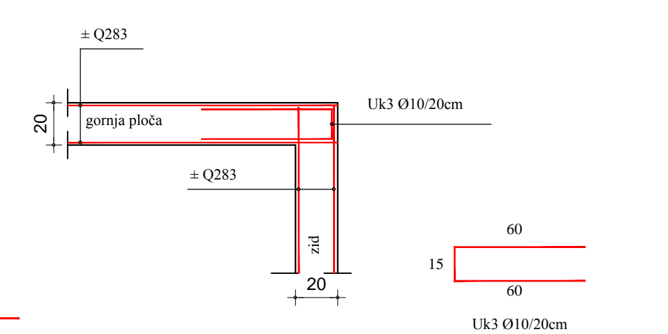
SPOJ GORNJE PLOČE I ZIDA ŠAHTA
