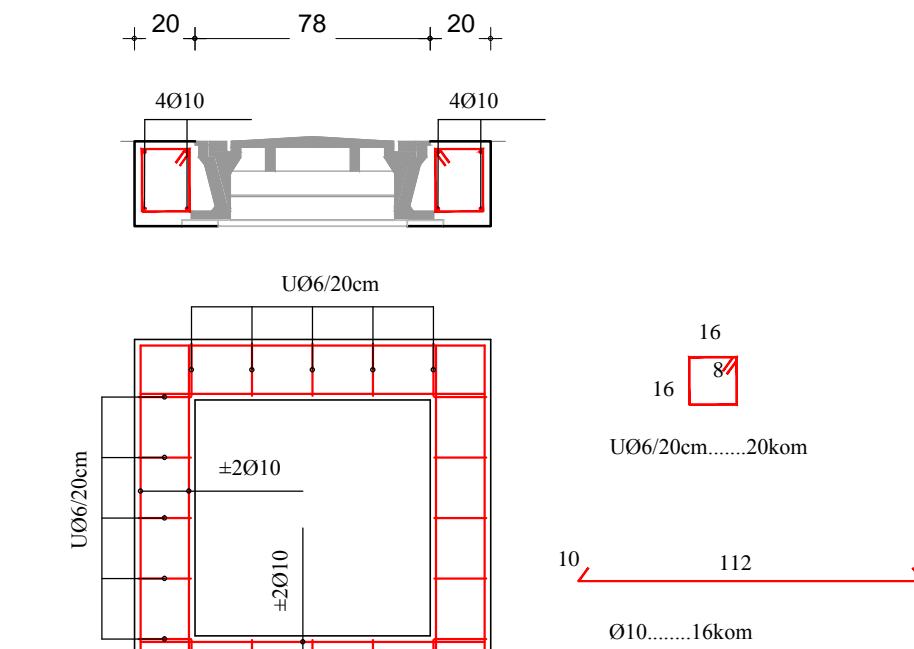
AB PRSTEN (KVADRATNI) 20/20cm
