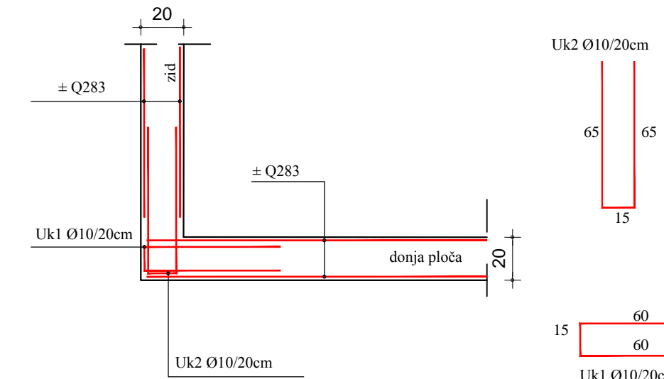
SPOJ DONJE PLOČE I ZIDA ŠAHTE
