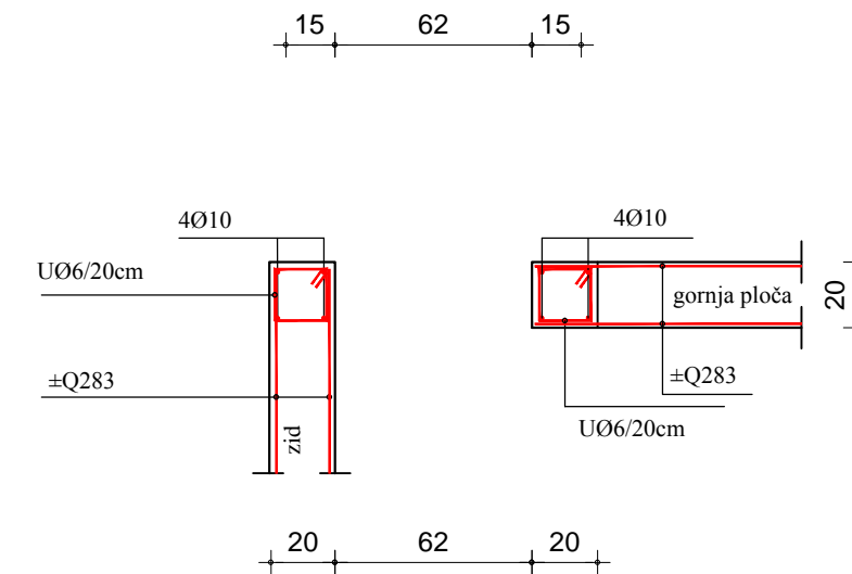
DETALJ SPOJA GORNJE PLOČE I ULAZA U ŠAHT
