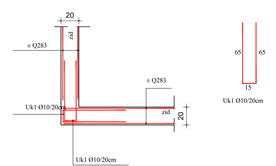
SPOJ ZIDOVA ŠAHTE
