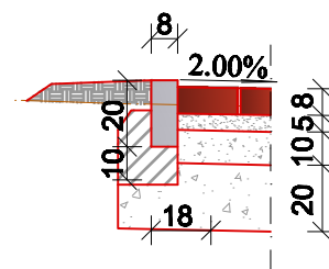
детал "А" ивичњак 8/20 R=1:25
