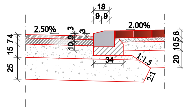
детал "Б" оборени ивичњак 12/18 R=1:25
