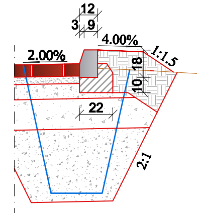
детал "В" ивичњак 12/18 R=1:25
