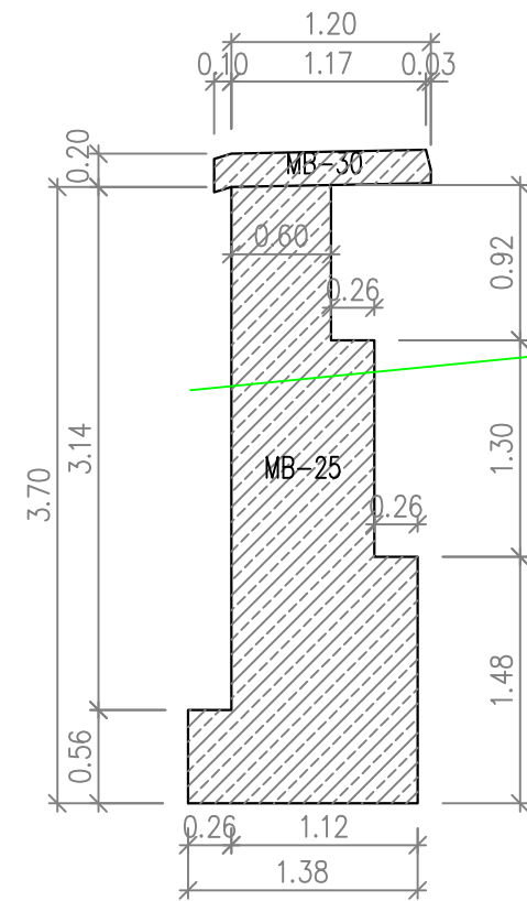
PRESEK 3-3
