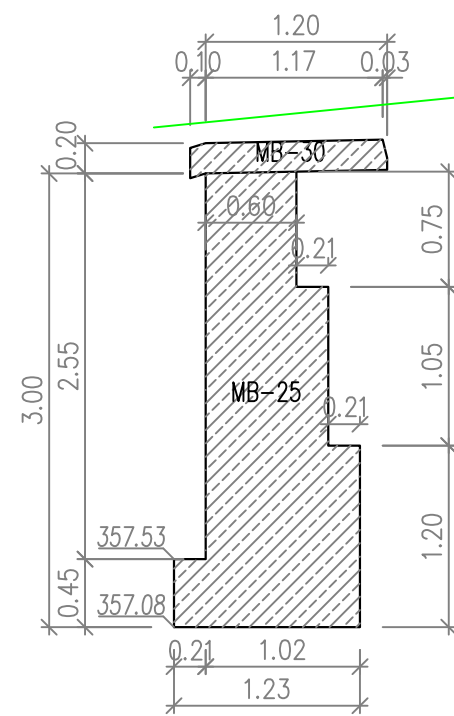
PRESEK 2-2
