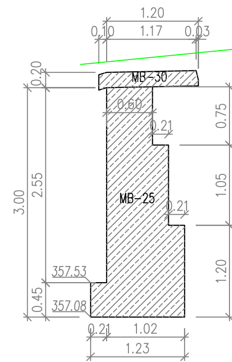
PRESEK 1-1
