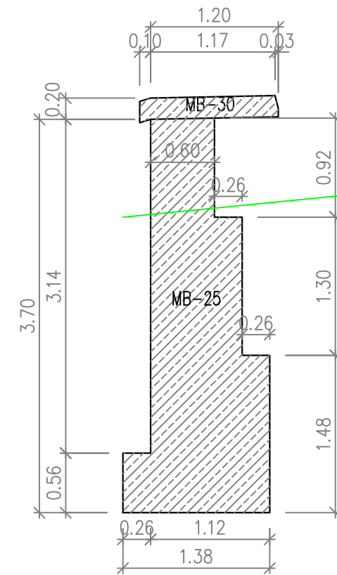
PRESEK 4-4
