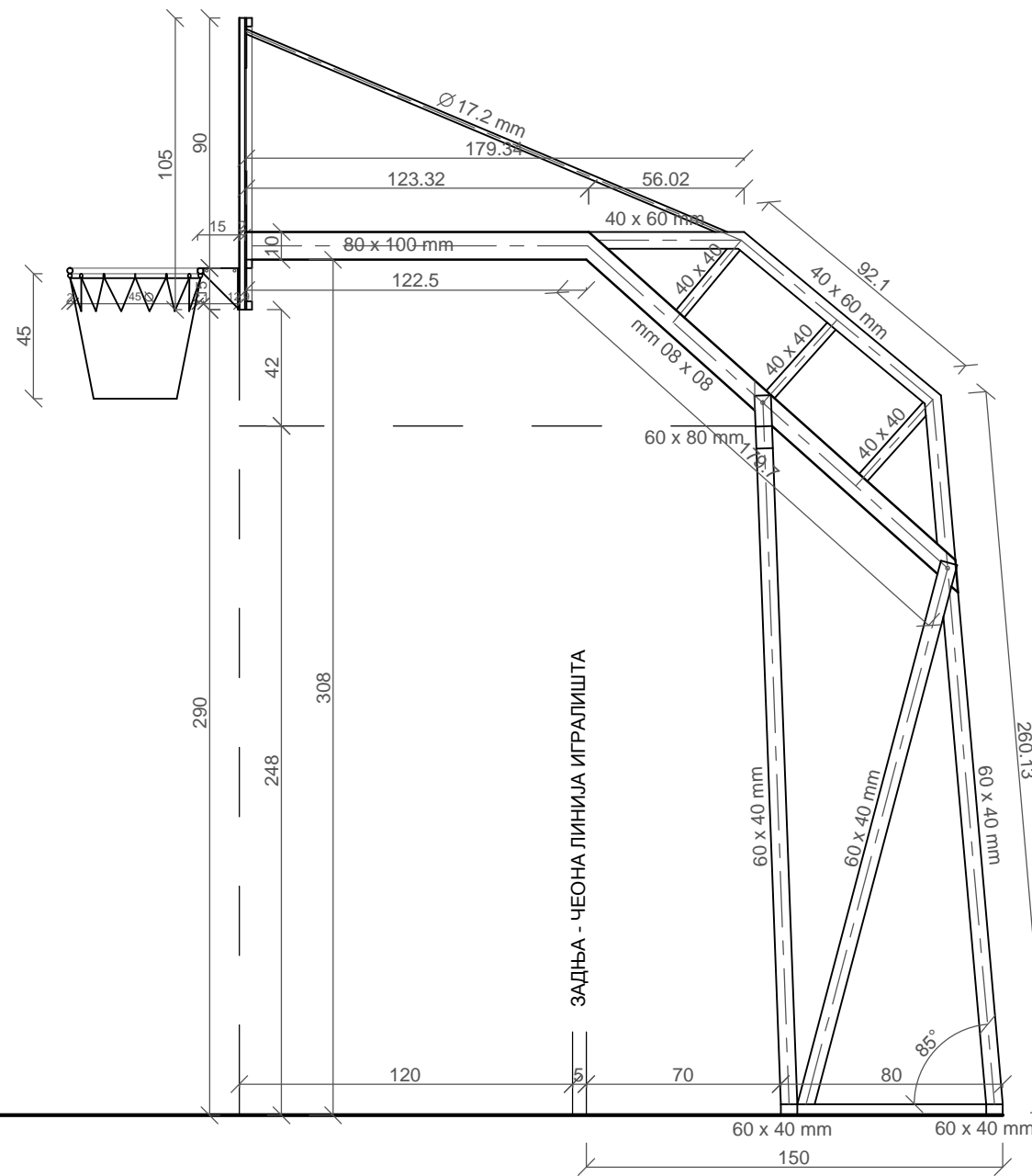
БОЧНИ ИЗГЛЕД ТАБЛЕ И КОША
