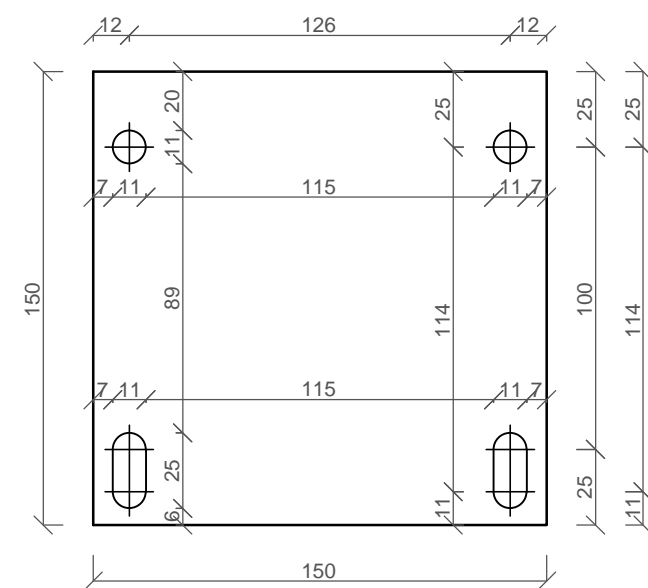
ИЗГЛЕД КОНТАКТНЕ ПЛОЧЕ (димензије у милиметрима)
