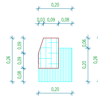
Детаљи малог ивичњака P=1:10
