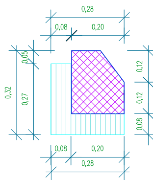
Детаљи ивичњака P=1:10
