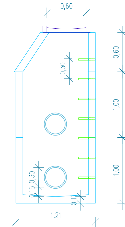
Детаљ шахте P=1:25
