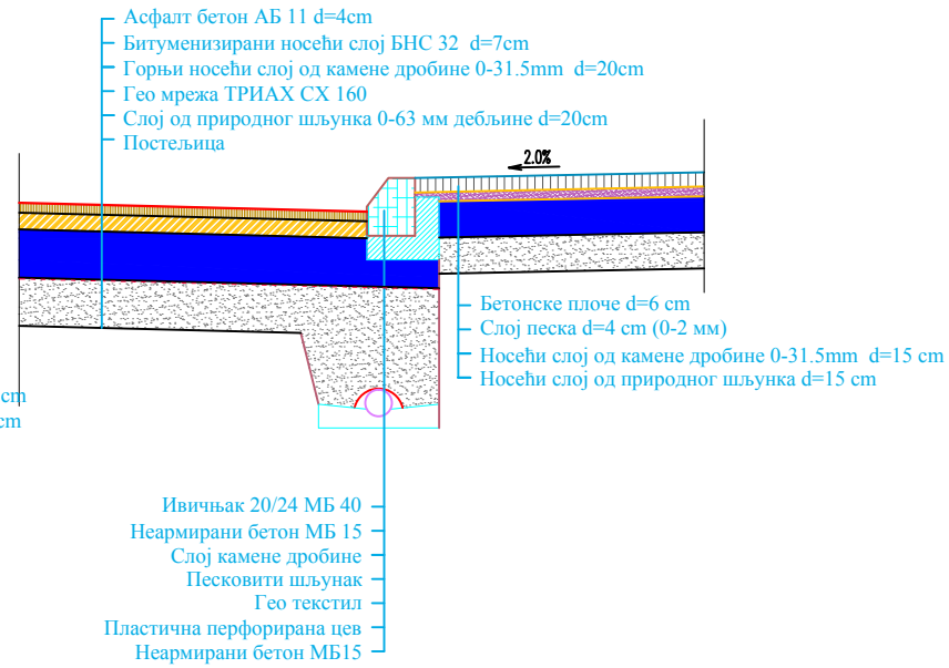
Детаљ дренаже P=1:25
