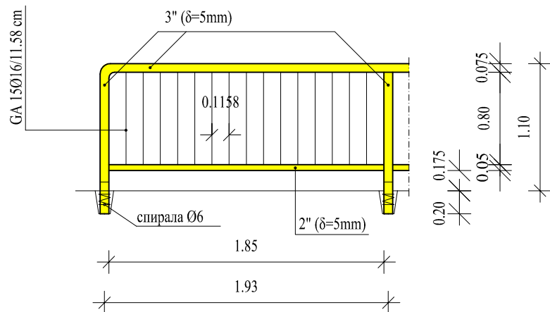
ДЕТАЉ -А- Р=1:25
