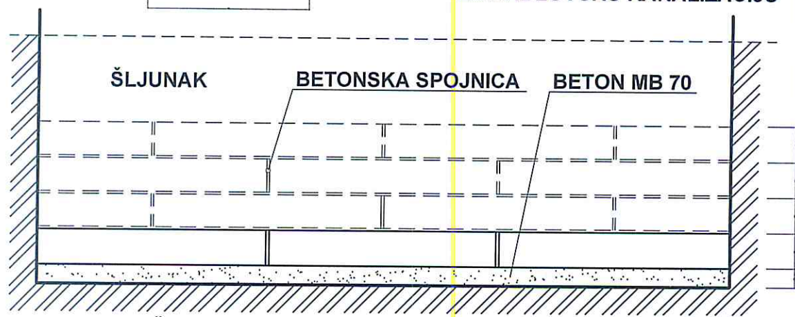
PODUŽNI PRESEK ROVA ZA KABLOVSKU KANALIZACIJU
