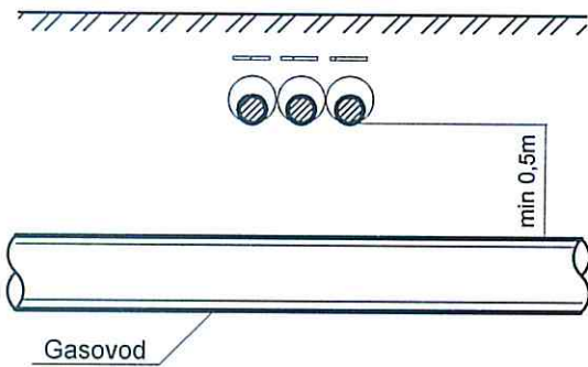
PRESEK 1 - 1
