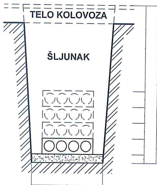
POPREČNI PRESEK ROVA ZA KABLOVSKU KANALIZACIJU
