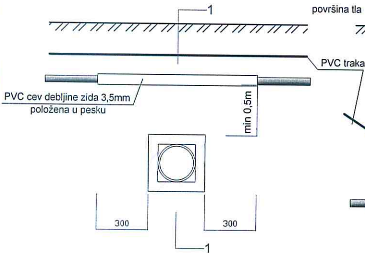
PRESEK 1 - 1
