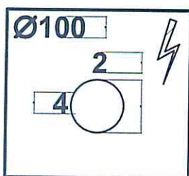
Kablovska kanalizacija Ø100 u 2 reda po 4 otvora
