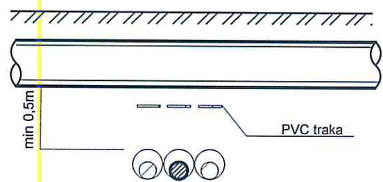
PRESEK 2 - 2
