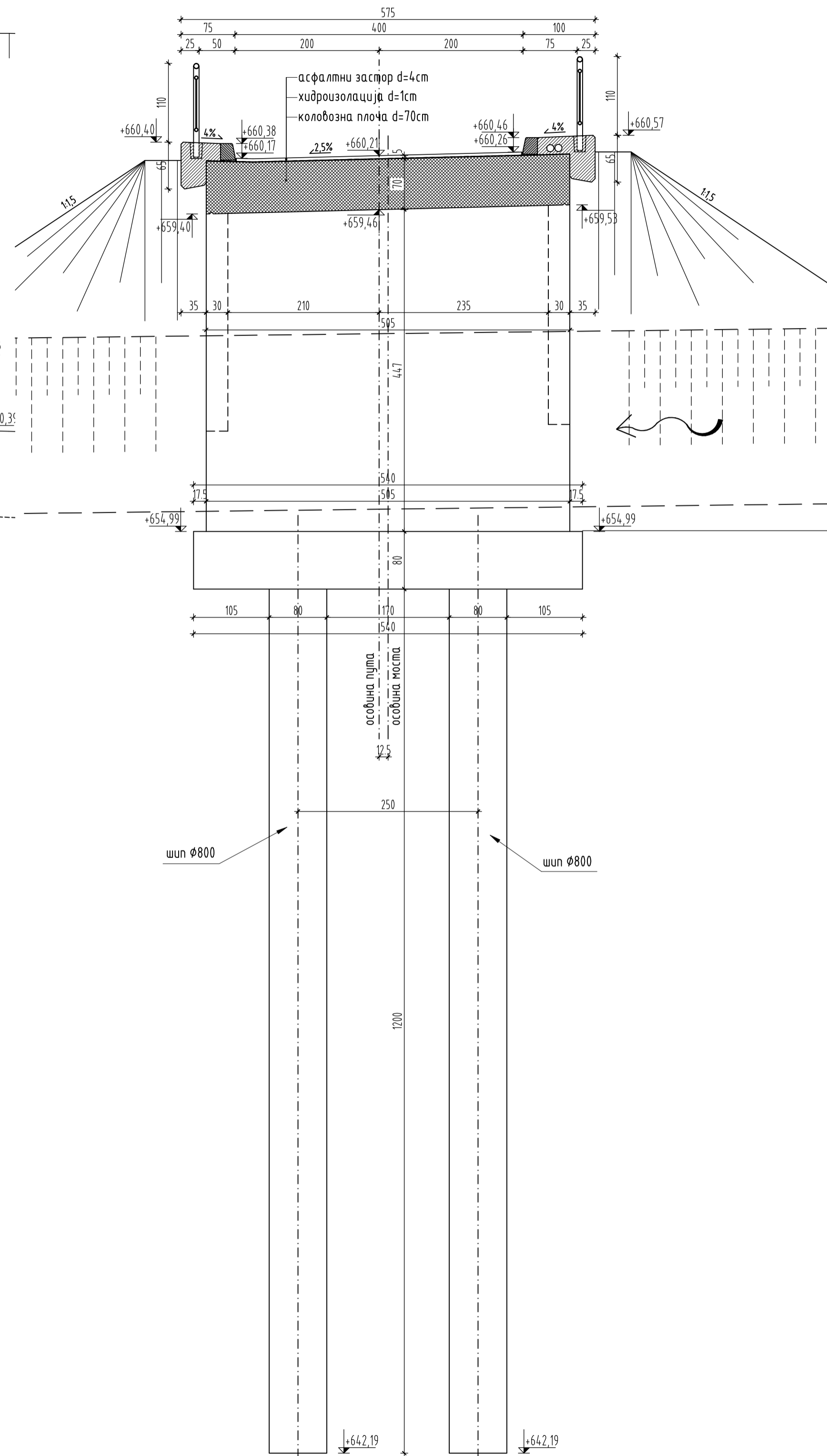
ПОПРЕЧНИ ПРЕСЕК 1:50
