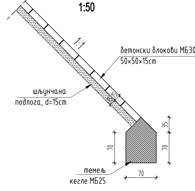
Темељ кегле 1:50
