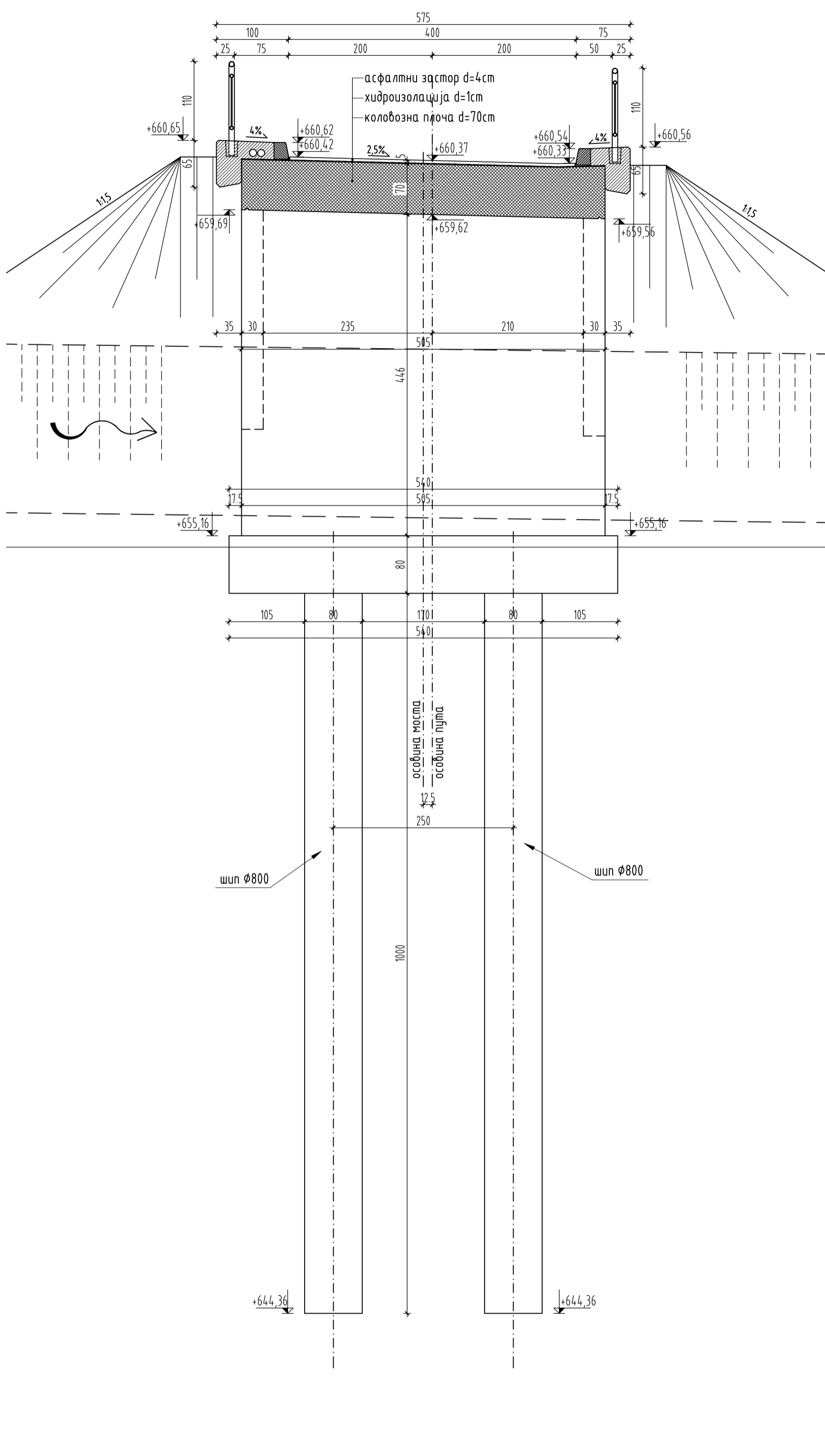
ПОПРЕЧНИ ПРЕСЕК 1:50
