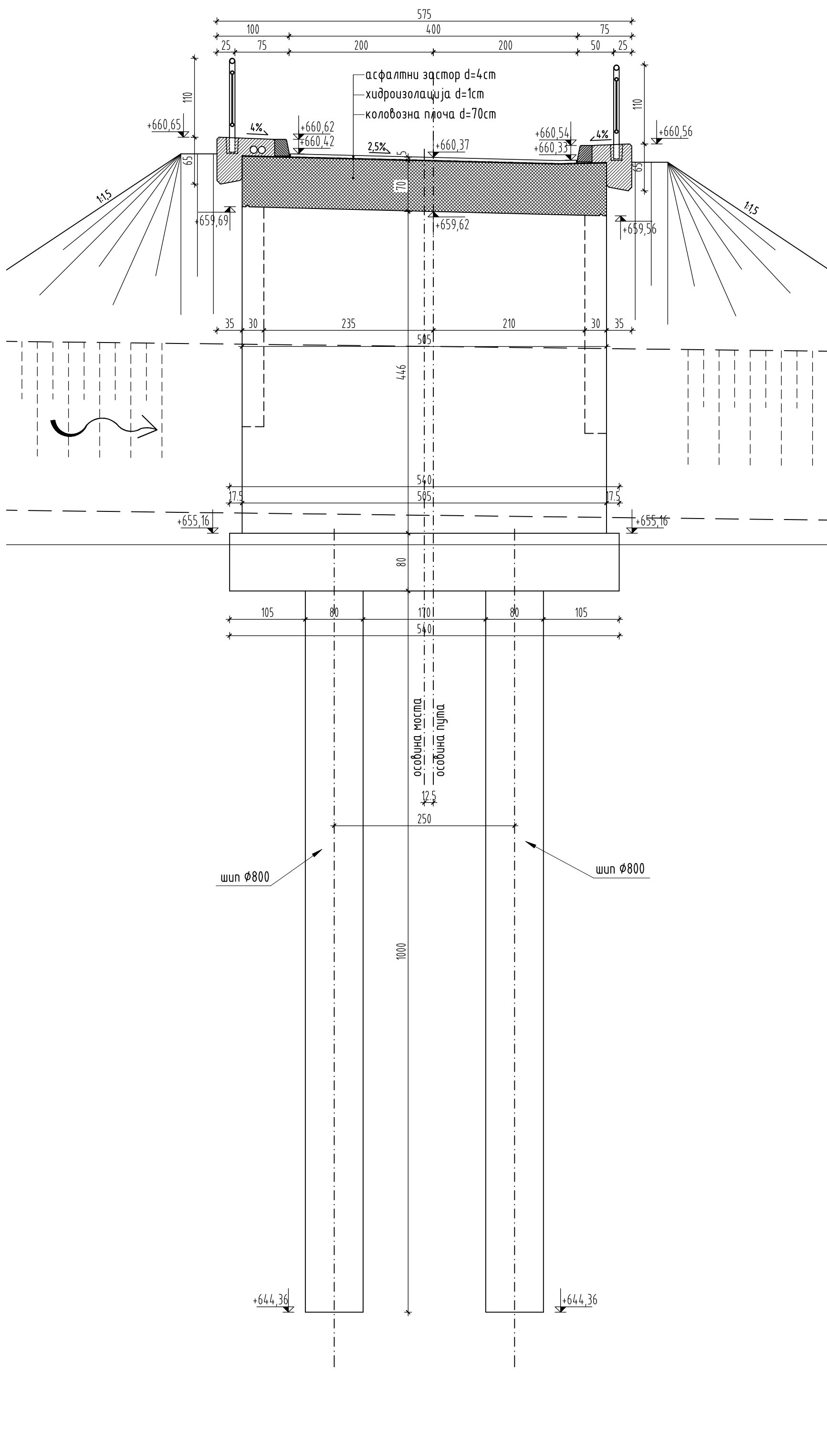
ПОПРЕЧНИ ПРЕСЕК 1:50
