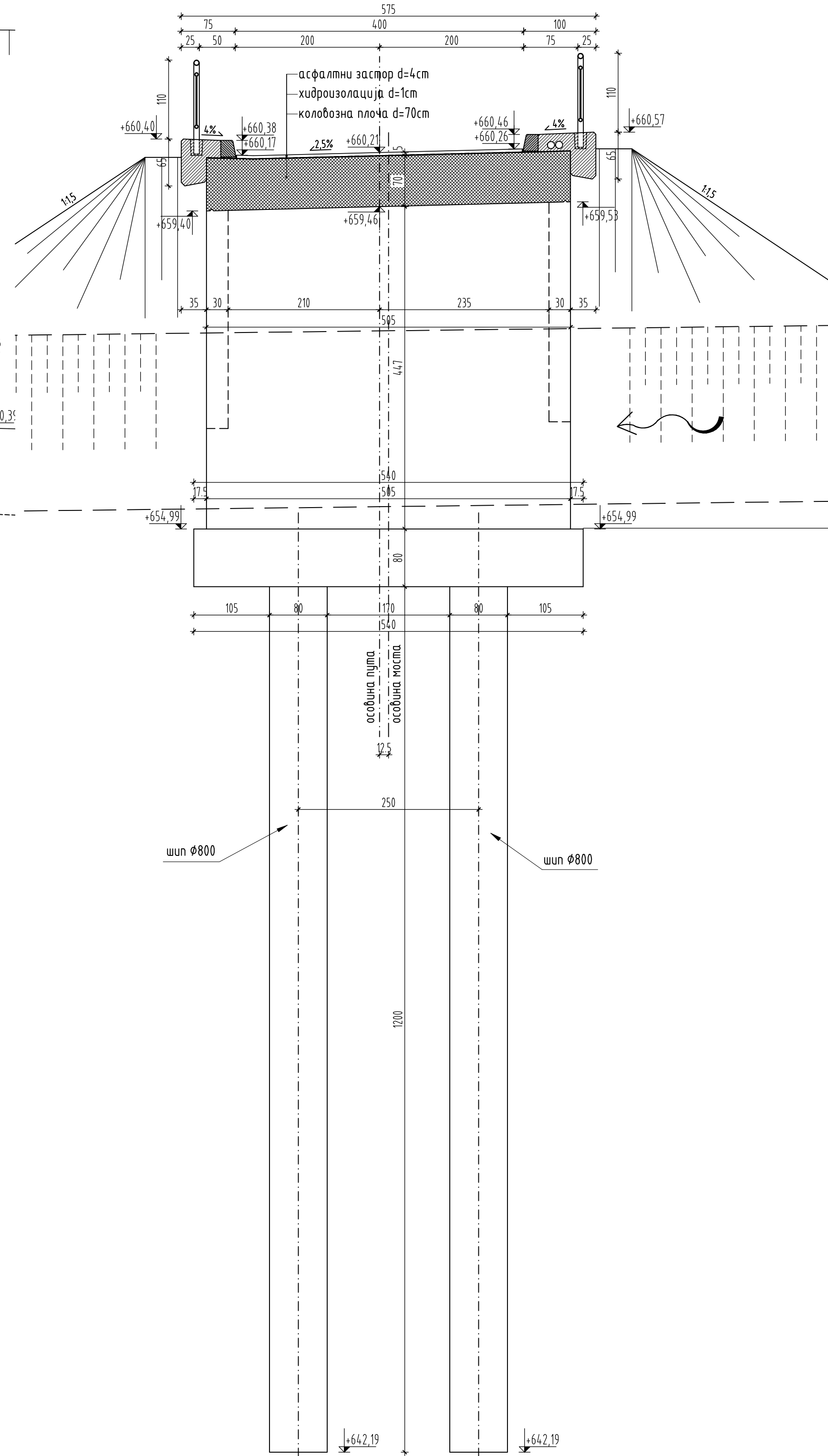
ПОПРЕЧНИ ПРЕСЕК 1:50
