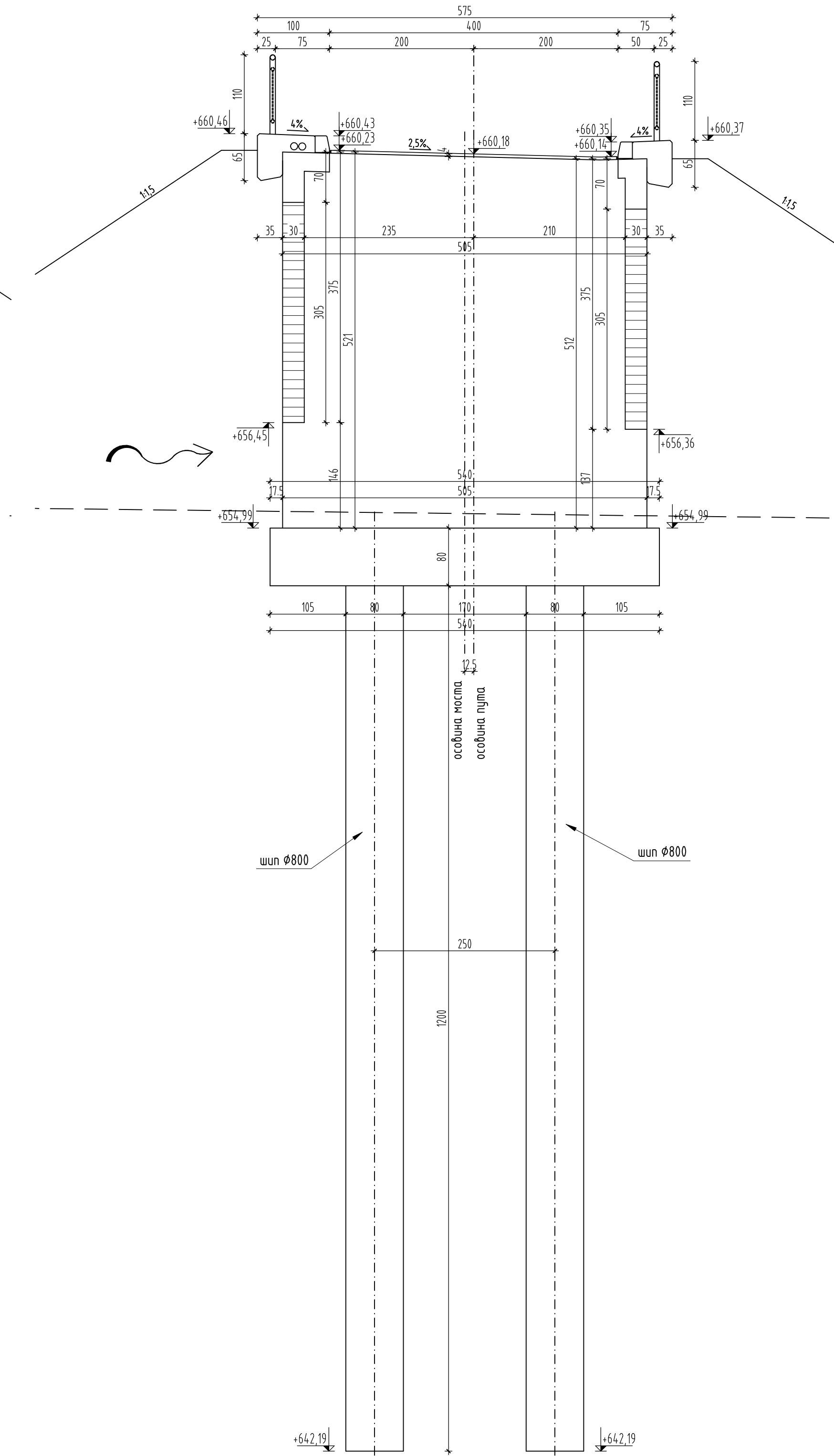
ПОПРЕЧНИ ПРЕСЕК 1:50
