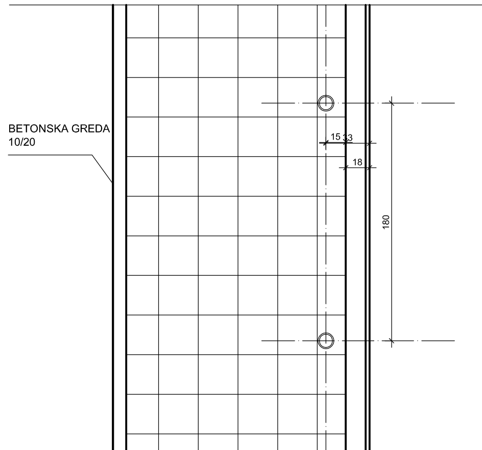
Osnova trotoara
