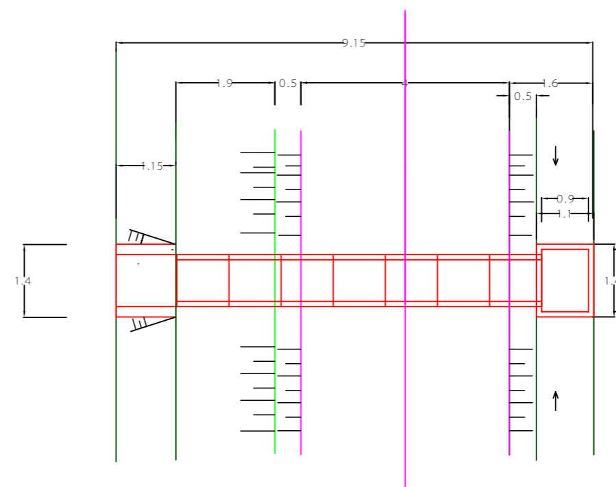
PODU@NI PRESEK "B - B" R=1:100
