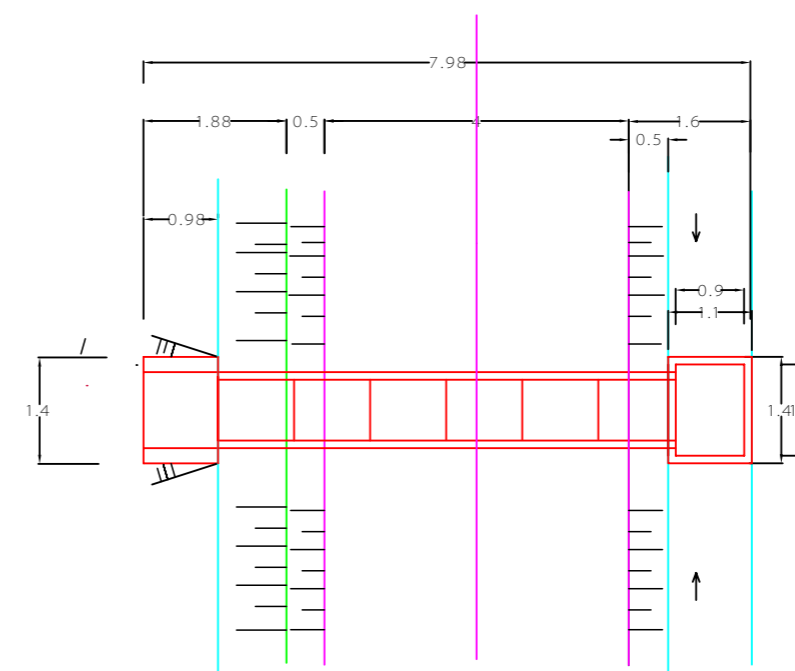
PODU@NI PRESEK "B - B" R=1:100
