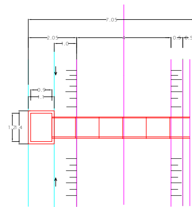
PODU@NI PRESEK "B - B" R=1:100
