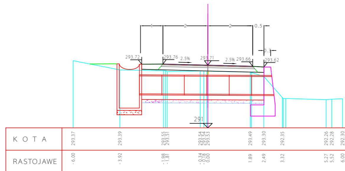
PODU@NI PRESEK "B - B" R=1:100
