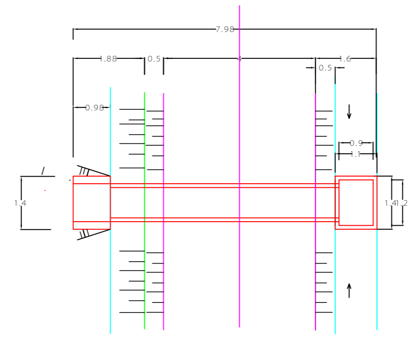
PODU@NI PRESEK "B - B" R=1:100
