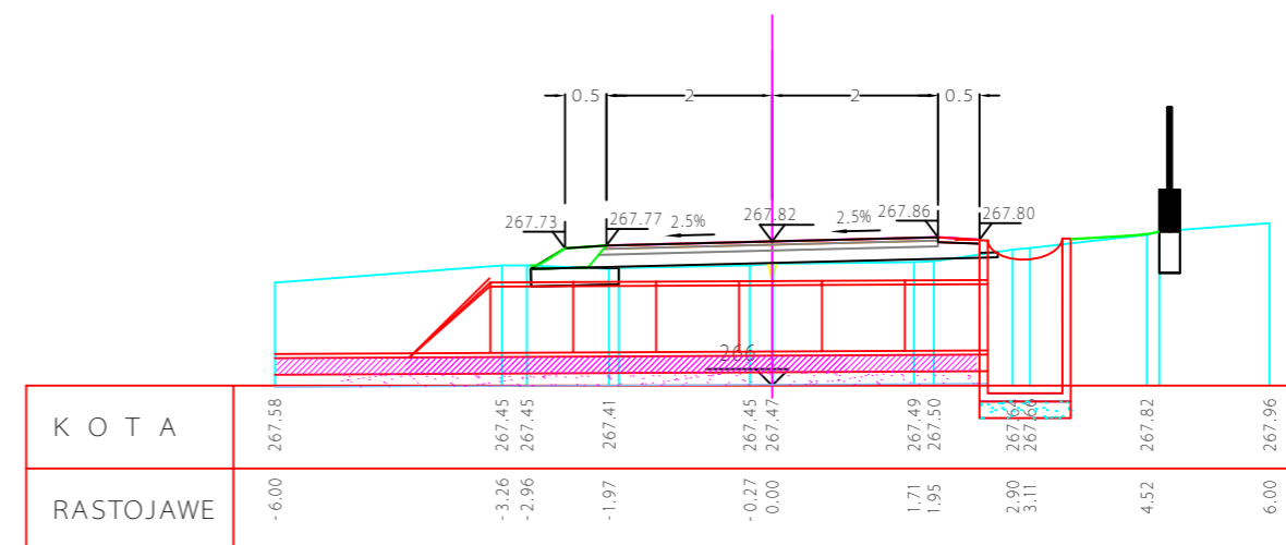
PODU@NI PRESEK "B - B" R=1:100
