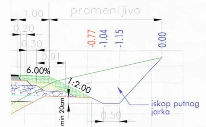
detalj bankine i putnog jarka R=1:50
