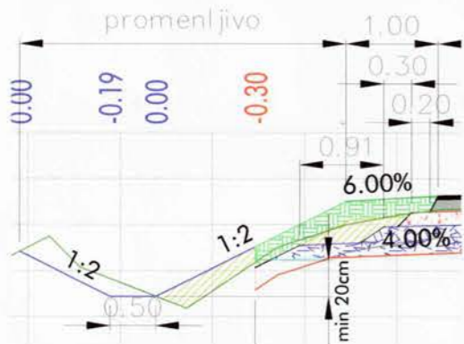
detalj bankine i putnog jarka R=1:50
