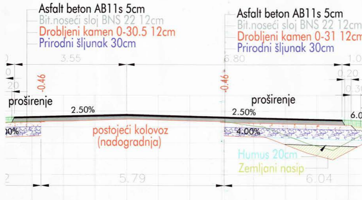
detalj kolovoza sa proširenjem R=1:50
